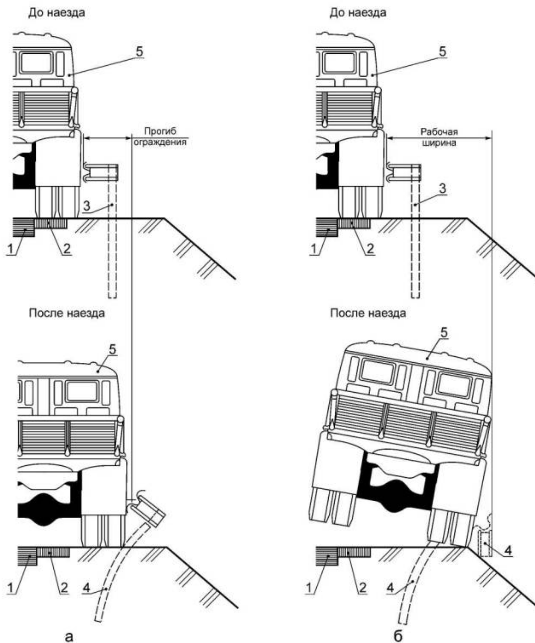
Рисунок В.24 - Пример размещения светофоров: а - на перекрестке; б - на разделительной полосе и над проезжей частью
