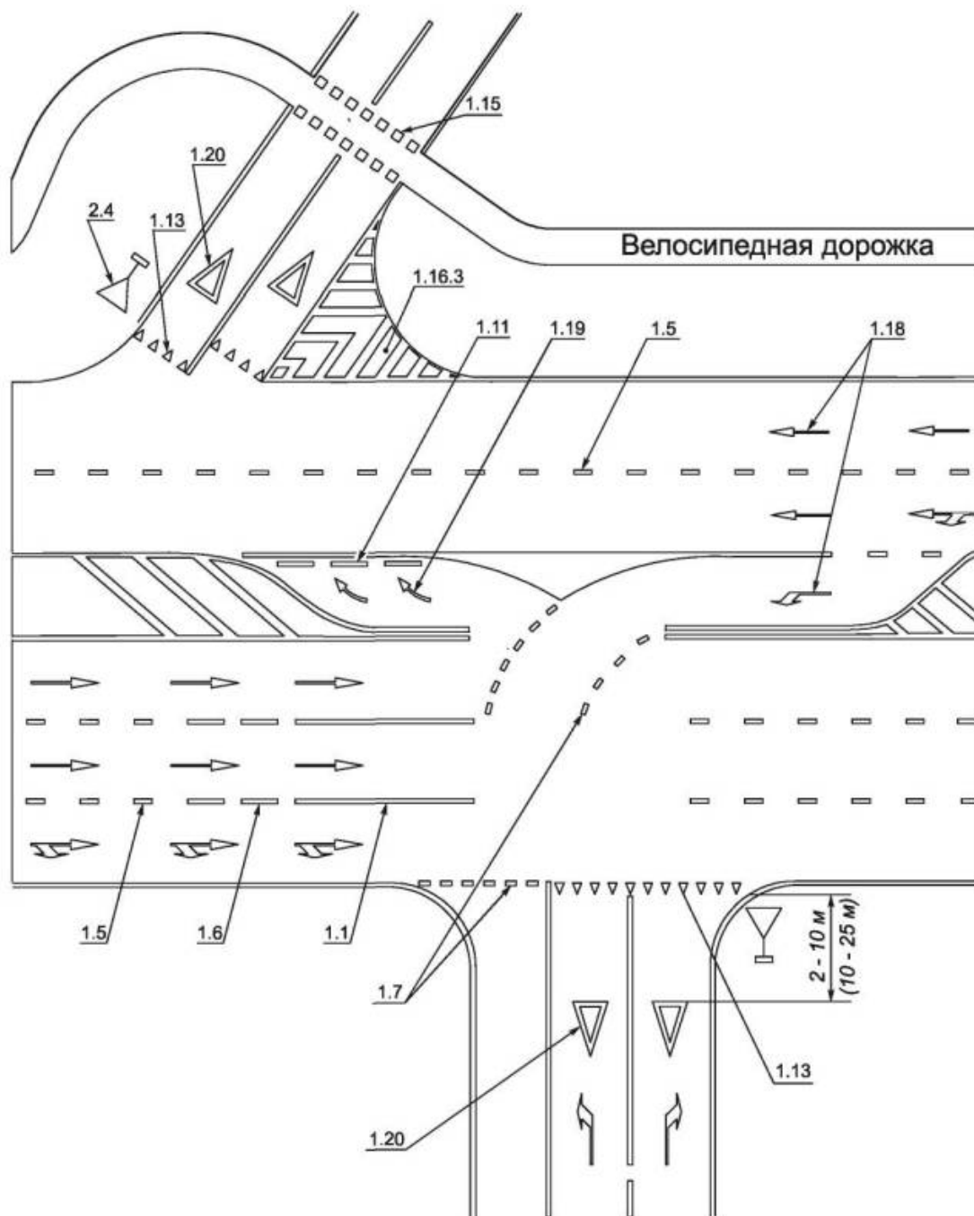
Рисунок В.10 - Пример нанесения разметки канализированного пересечения
