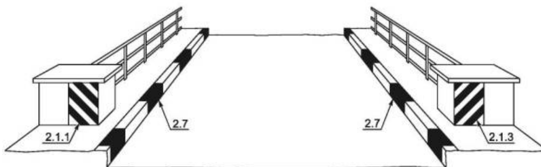
Рисунок В.21 - Пример нанесения разметки 2.1.1, 2.1.3 и 2.7
