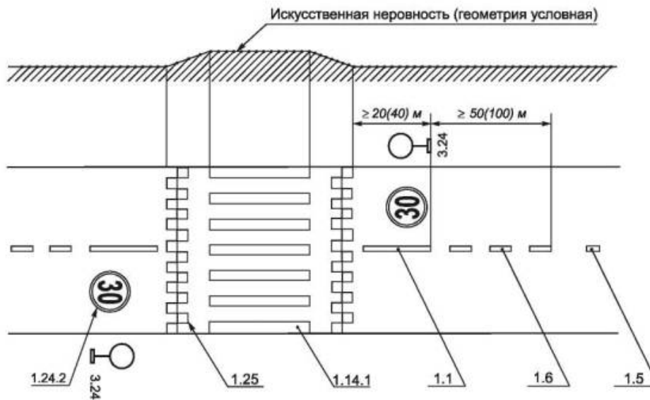
Рисунок В.19 - Пример нанесения разметки 1.25
